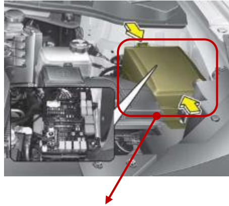
PE(Engine) room fuse box
