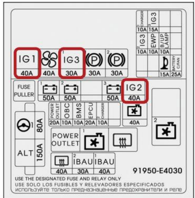
PE(Engine) room fuse box
